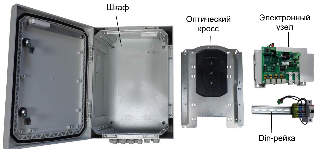
Рисунок 3.1.3 – Основные элементы коммутатора
