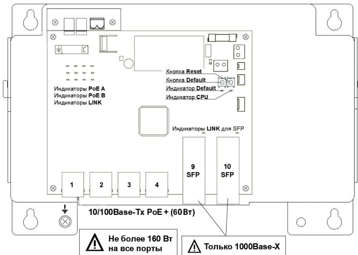
Рисунок 3.4.2 - Расположение элементов PSW-2G+Box
